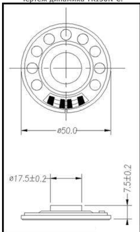
Чертёж динамика TRI50N-C:
